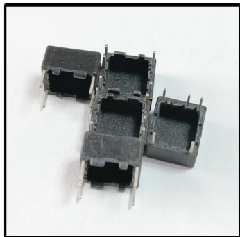
变压器壳检测
