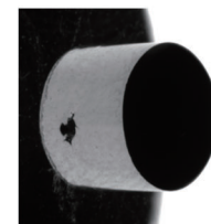
车床件检测平面毛刺 侧面高度、平行度
