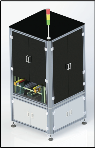
底部避空双边输送在线检测机
